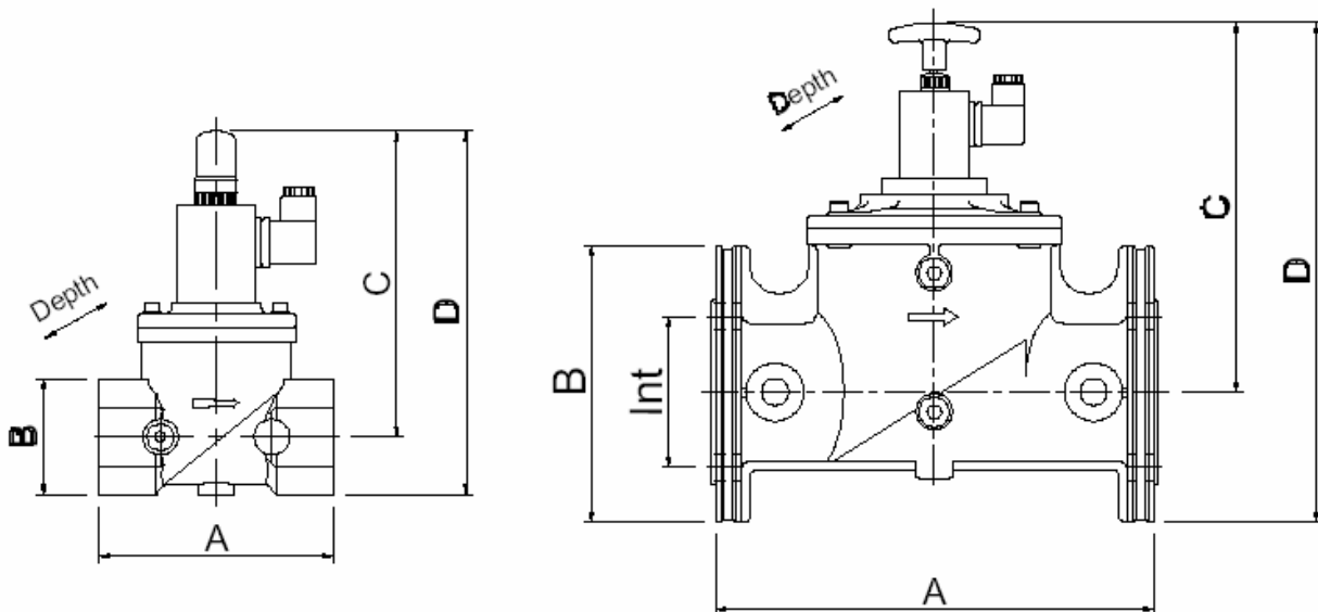
Размеры, мм (для моделей до 6 бар маркировка EVRM6NC...)
