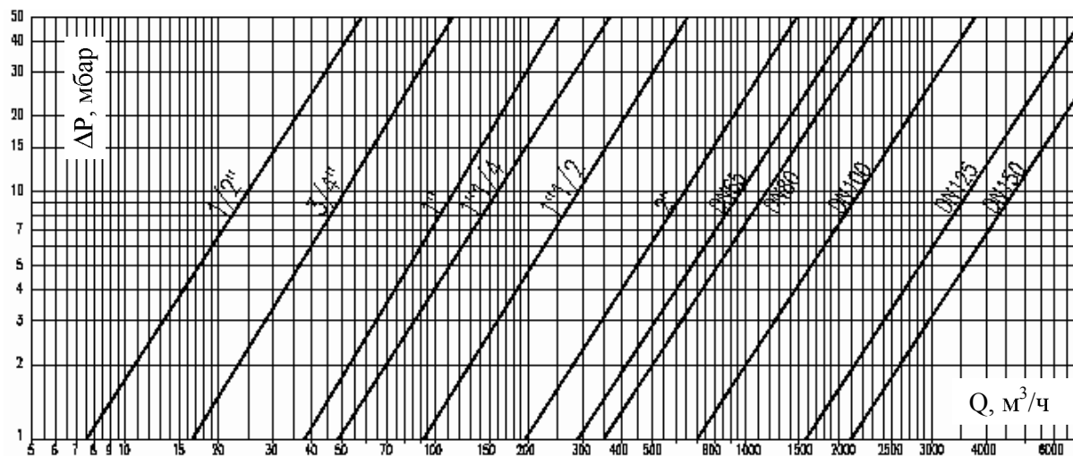
Диаграмма зависимости потери давления \Delta P от расхода Q (для природного газа, н.у.)
