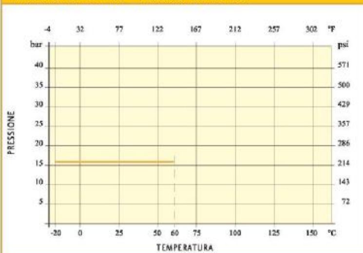
PRESSIONE/TEMPERATURA - PRESSURE/TEMPERATURE
