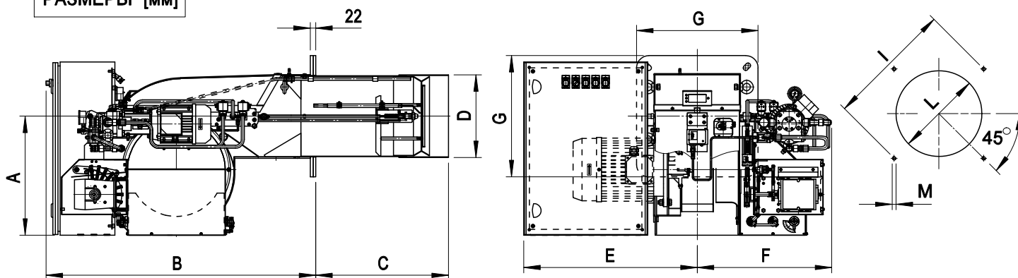
РАЗМЕРЫ [мм]
