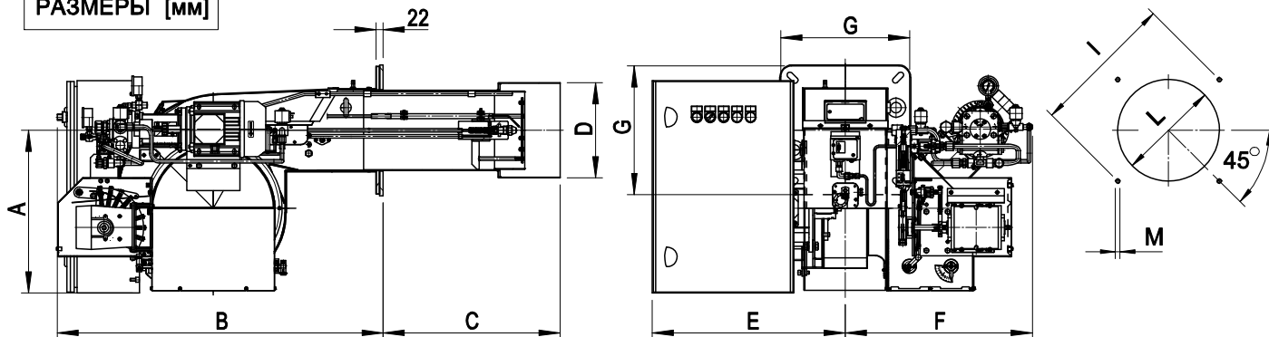
РАЗМЕРЫ [мм]
