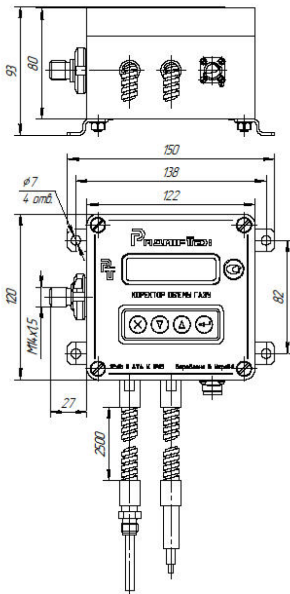
Рисунок А.1 – Габаритні та приєднувальні розміри коректора ВЕГА-1.01 без вбудованого GSM модема
