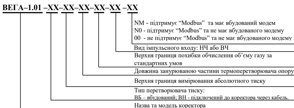
Рисунок 1 – Схема складання умовного позначення коректору ВЕГА-1.01
