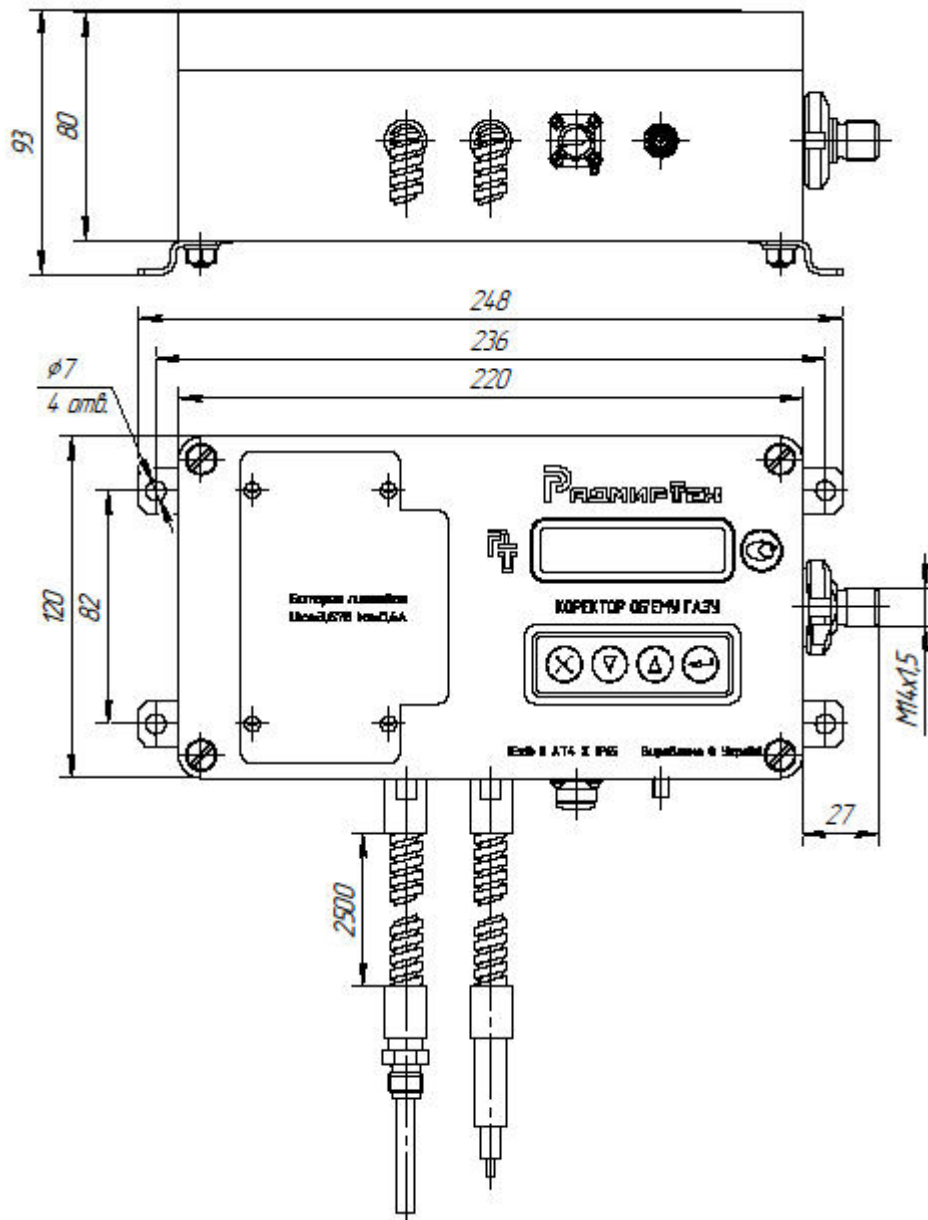
Рисунок А.2 – Габаритні та приєднувальні розміри коректора ВЕГА-1.01 з вбудованим GSM модемом
